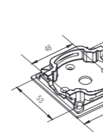
Schnellmontagelager 10Nm - 30Nm ID 413
