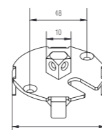
Vierkantlager 10x10mm ID 555
