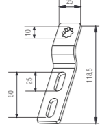
Fertigkastenlager m. Sternaufnahme ID 259
