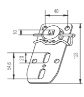
Fertigkastenlager m. Abrollfunktion ID 280
