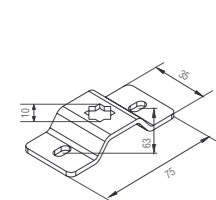
Sterngegenlager ID 554
